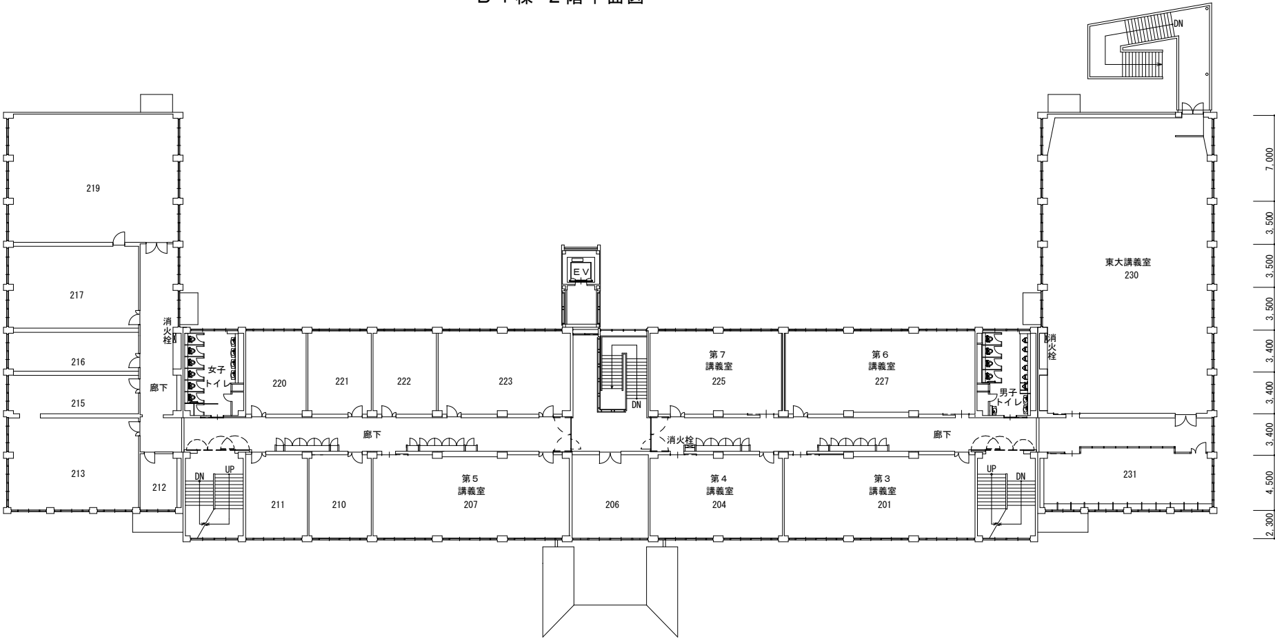
B 1 棟 2 階平面図
